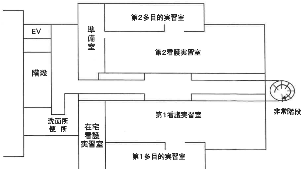
4階平面図
