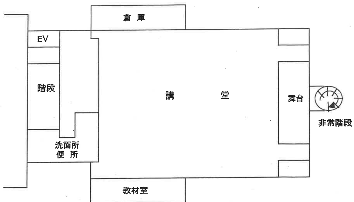
7階平面図
